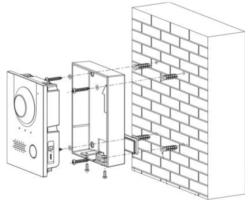
Montaje empotrado
