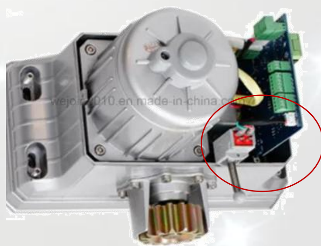
Se instala en la placa del motor con 2 tornillos y se conecta a la controladora
