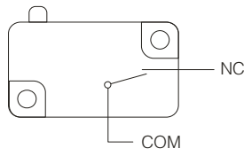
常闭型 SPST-NC(1B)
