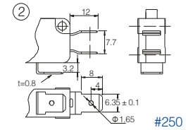
常开型 SPST-NO(1A)
