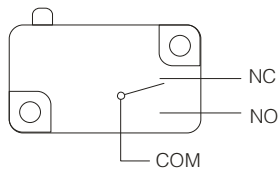
双投型 SPDT(1C)
